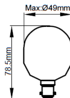
P45-B15(IEC60630)
