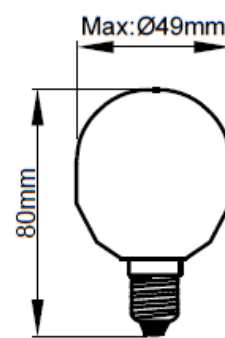
P45-E14(IEC60630)
