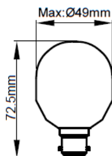
P45-B22(IEC60630)
